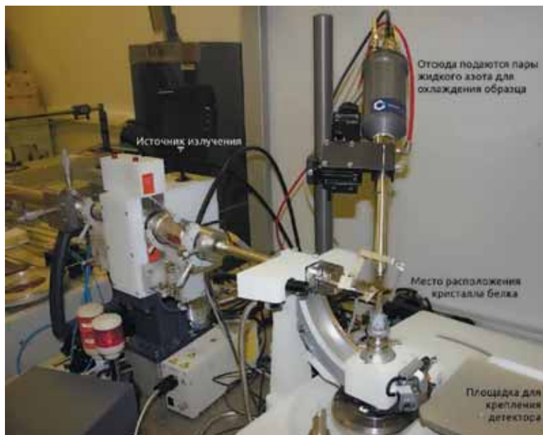
Установка крупным планом. Оранжевые и красные индикаторы загораются при работе, а сама установка смонтирована за специальным стеклянным ограждением для защиты персонала от облучения
