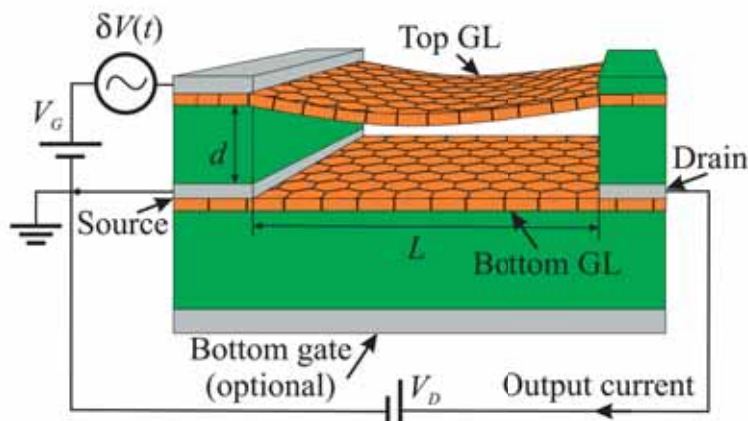
Схема детектора
