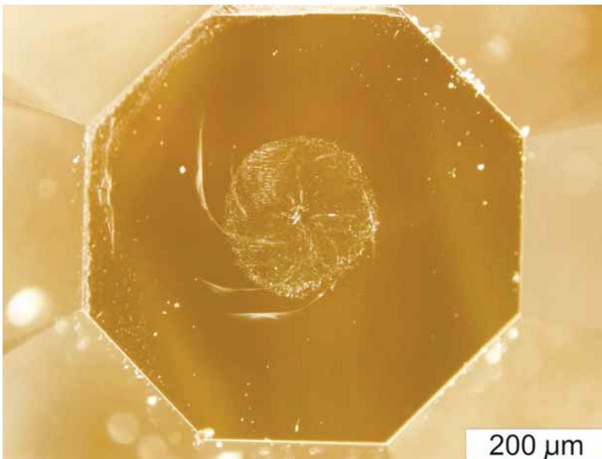
Алмазные наковальни, повреждённые во время синтеза фуллеритов. Обратите внимание на вмятину в центре
